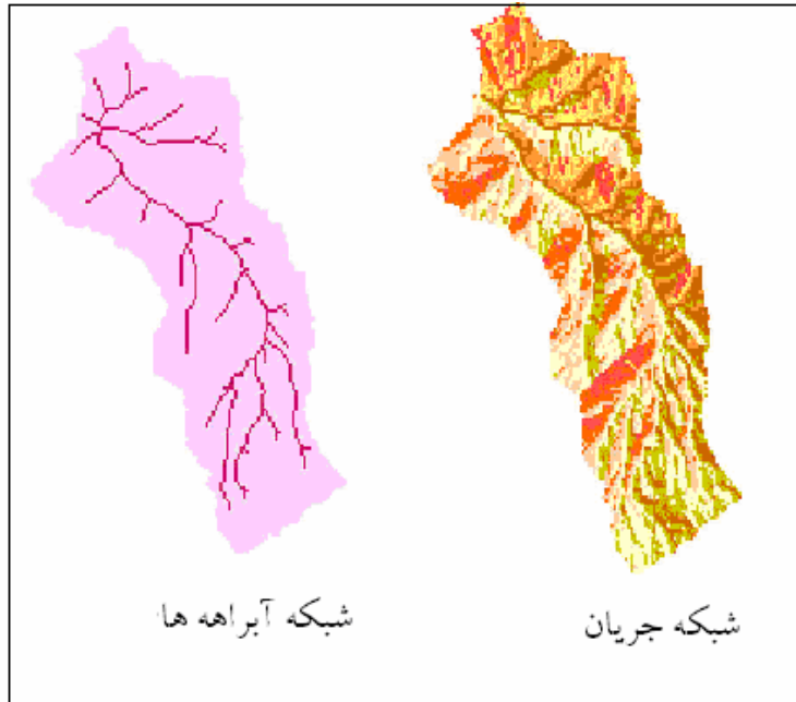
شکل ۳- ترسیم شبکه‌ی جریان و شبکه‌ی آبراهه‌های حوضه‌ی آبخیز کسلیان با استفاده از برنامه‌ی HEC-Geo HMS.
