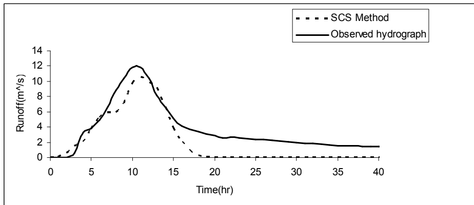
شکل ۹- اعتباریابی شبیه‌آشناسی حوضه‌ی آبخیز کسلیان با مقایسه‌ی آب‌نگار شبیه‌سازی شده با کاربرد شبیه SCS و آب‌نگار واقعی سیلاب ۲۲ اکتبر ۱۹۹۴.
