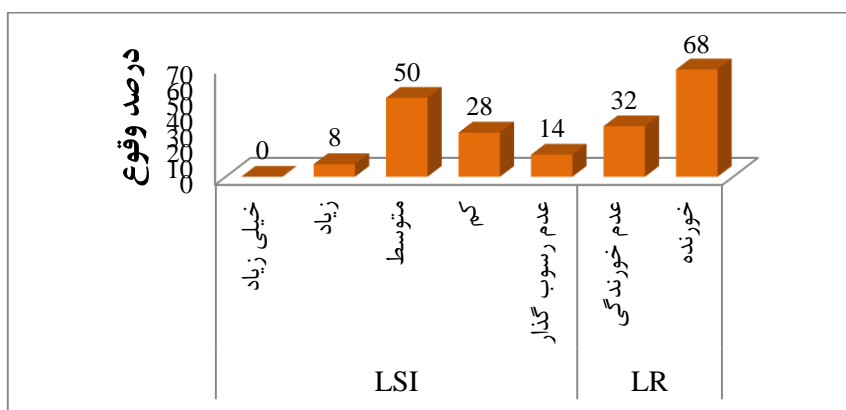
شکل ۸- درصد وقوع وضعیت های مختلف شاخص های خورندگی و رسوب گذاری آب زیرزمینی
