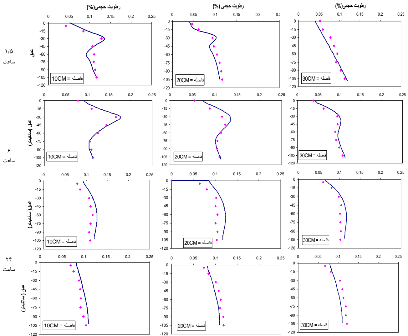
شکل ۱- مقایسه ی درصد های رطوبت شبیه سازی شده و مشاهداتی در زمانهای ۱/۵ و ۶ ساعت هنگام آبیاری ، و ۲۴ و ۹۶ ساعت بعد از آبیاری (• مقادیر مشاهداتی، — مقادیر شبیه سازی شده).
