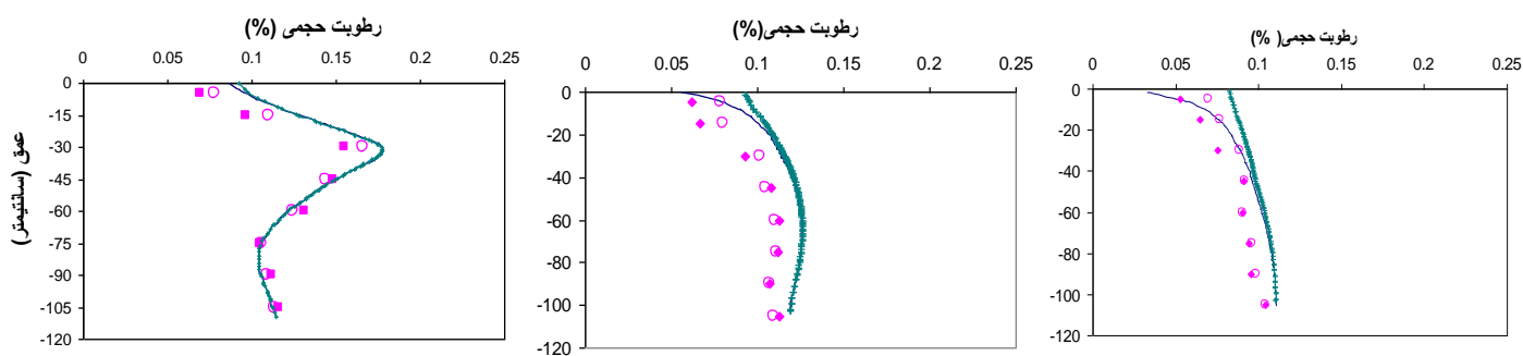
شکل ۴ - مقایسه ی تاثیر خاکپوش بر الگوی رطوبت به ازاء کاربرد بده ی ۲ لیتر بر ساعت (شبیه با خاکپوش +، مشاهده بدون خاکپوش ■، مشاهده با خاکپوش ○. مدل بدون مالچ —)
