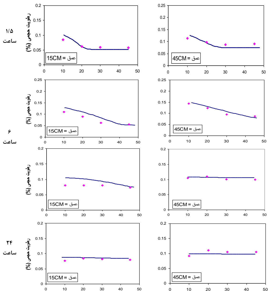
شکل ۲- مقایسه ی درصد های رطوبت شبیه سازی و مشاهداتی در عمقهای ۱۵ و ۴۵ سانتیمتری، و در زمانهای ۱/۵ و ۶ ساعت هنگام آبیاری، و ۲۴ و ۹۶ ساعت بعد از آبیاری (♦ مقادیر مشاهداتی، — مقادیر شبیه سازی شده)
